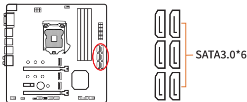
图2 -11 SATA接口
