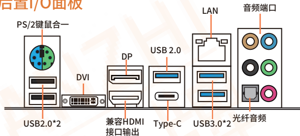
图1-2 整体后置I/O面板展示
