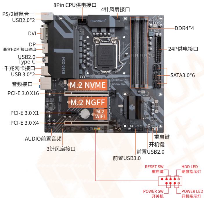
图1-1 B360-ZD4 V1.0主板图解
